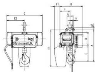
Versión de 1 ramal de cadena
