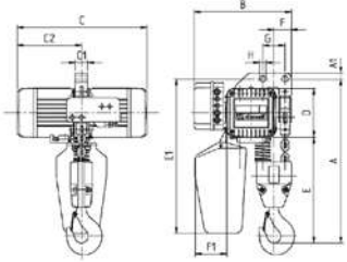
Versión de 2 ramales de cadena
